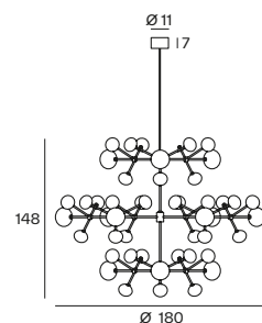
552.48L Chandelier
