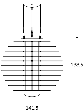
0024/3VN ø 141,5 x 138,5 4x54W (FL) G5
