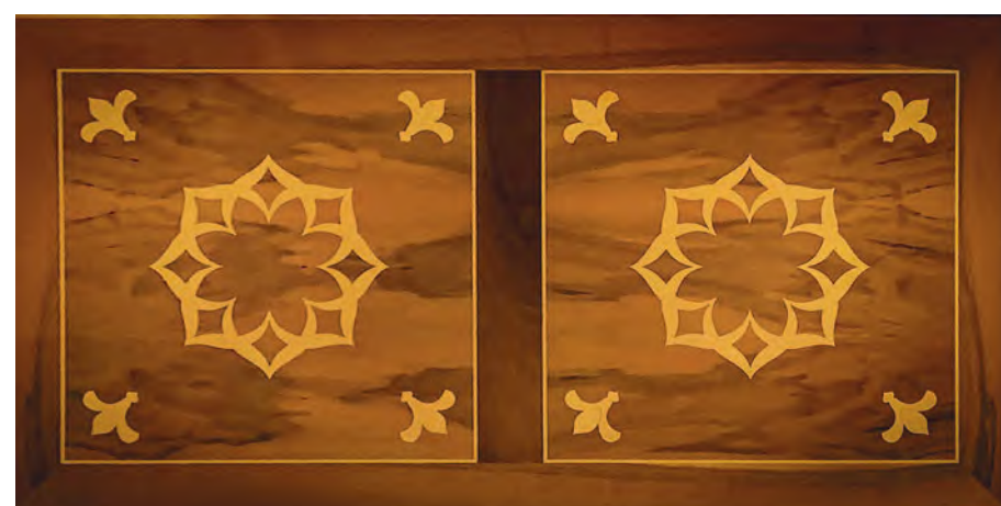
ARTICOLO | H512 Tavolo allungabile con intarsio Giglio e 2 allunghe da cm. 40, gamba nr. 20 Extension table with Giglio inlay and 2 leaves cm. 40, legs nr. 20 cm. L. 170 P. 90 H. 79 (aperto L. 250 P. 90) M3 0,28 Kg. 59
