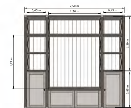
ARTICOLO| H650 Parete con luci led con 2 porte e 2 cassetti. Composition 2 doors and 2 drawers with led. cm. L. 250 H. 225 P. 43 M3 0,6 smontata Kg. 190
