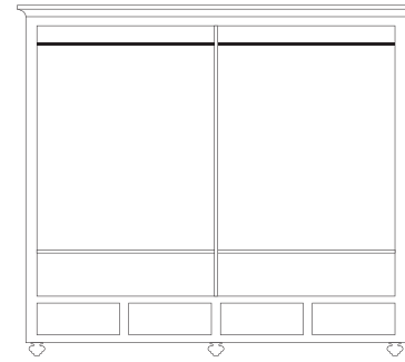
458/A Armadio 4 a. 4 c. smontabile Detachable wardrobe L 250 P 63 H 220 Finitura P11
