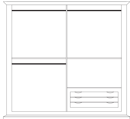
2166/A Armadio 2 a. scorrevoli smontabile con cassetiera Detachable wardrobe chest of drawers included L 275 P 66 H 254 Finitura RAL 7047 con profili P04
