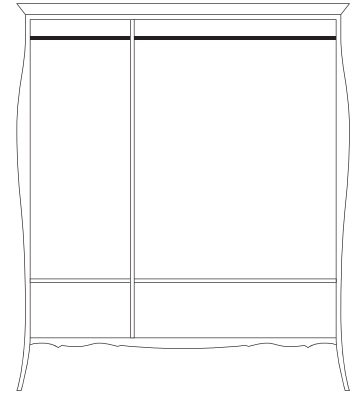
492/A Armadio 3 a. smontabile Detachable wardrobe L 182 P 64 H 212 Finitura P09.02
