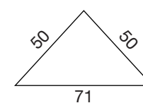
724/A Angolo 1 p. 1 c. Corner cabinet Lato 50 H 130 Finitura P01
