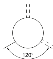
COS.CON.1 Rosone per Driver da 1 a 6 luci (da 1 a tre bracci) Ø20 - H 4.5 cm Canopy for drivers with 1 to 6 lights (1 to 3 arms) Ø20 - H 4.5 cm
