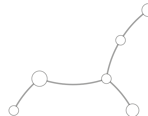
COSTELLAZIONE 6 LUCI / 6 LIGHT COSTELLATION 3x COS.LP.1 1x COS.LP.2 1x COS.LP.2.LIN 1x COS.LP.3 3x COS.AJ.1 3x COS.AJ.3 3x COS.GLASS.16 2x COS.GLASS.21 1x COS.GLASS.25
