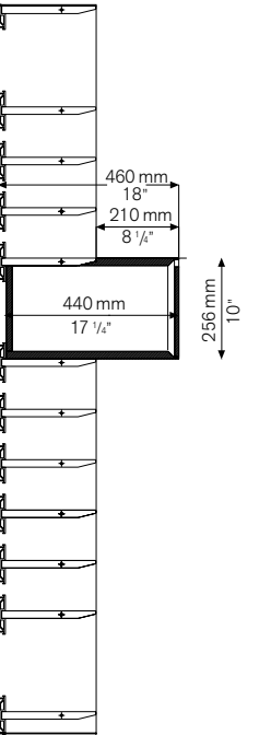
Elemento sporgente con cassetto posizionabile sospeso / Projecting element with drawer positionable sospeso
