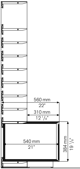
Elemento sporgente con cassetto anta ribalta posizionabile a terra / Projecting element with drawer flap door positionable on floor
