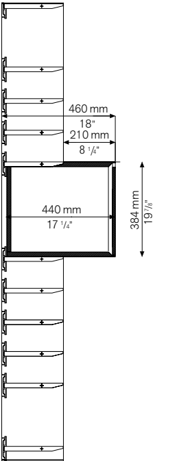
Elemento sporgente con anta a ribalta posizionabile sospeso / Projecting element with flap door suspended position
