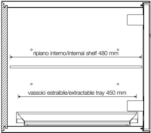
CONTENITORI STANDARD (profondità totale 550 mm) STANDARD STORAGE UNITS (total depth 550 mm)
