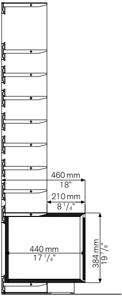
Elemento sporgente con anta ribalta posizionabile a terra / Projecting element with flap door positionable on floor
