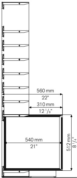
Elemento sporgente con anta complanare posizionabile a terra / Projecting element with flush sliding door positionable on floor
