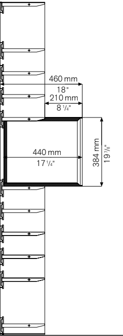
Elemento sporgente a giorno posizionabile sospeso / Open projecting element suspended position
