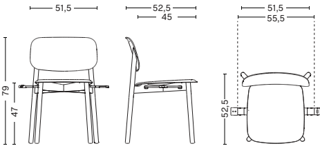
W51,5 X D52,5 x H79 cm Seat height 47,5 cm | Seat depth 44 cm
