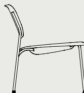
SOFT EDGE 100 W57 x D64 x H69/SH40 cm
