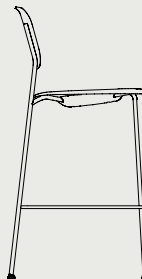
SOFT EDGE 90/95 HIGH W55 x D55,5 x H108/SH75 cm
