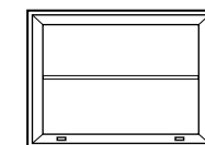
654/T Pensile vasistas / Wall unit L. 120 P. 40 H. 75,4
