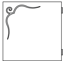
art. 51DX Anta push pull con rilievo / Door 63x63 sp. 1,8
