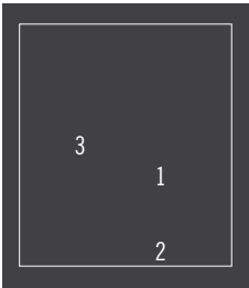
1 2095/3/AP/CR - 2095/3/AP/CR/CP - 2095/3/AP/CR/SP H min cm 25 - L cm 45 - Sp cm 12 - 3 G9 x 40W- Sp E14 x 60W - CP 3 E14 x 60W 2 2095/1/AP/CR - 2095/1/AP/CR/CP - 2095/1/AP/CR/SP H min cm 28 - L cm 12 - Sp cm 12 - 1 G9 x 40W- Sp 1 E14 x 60W - CP 1 E14 x 60W 3 2095/2/AP/CR - 2095/2/AP/CR/CP - 2095/2/AP/CR/SP H min cm 20 - L cm 40 - Sp cm 12 - 2 G9 x 40W- Sp 2 E14 x 60W - CP 2 E14 x 60W
