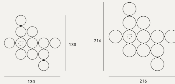
12 Elements-Ø23,5/Ø40
