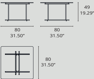
4230/1 V2 MESA | TABLE
