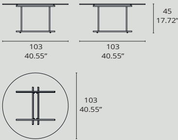
4230/1 V1 MESA | TABLE
