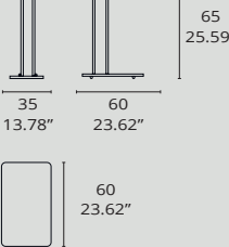
4230/3 V2 MESA | TABLE
