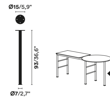
LEG solo per top con sbalzo > 50 cm only for tops with an overhang > 50 cm
